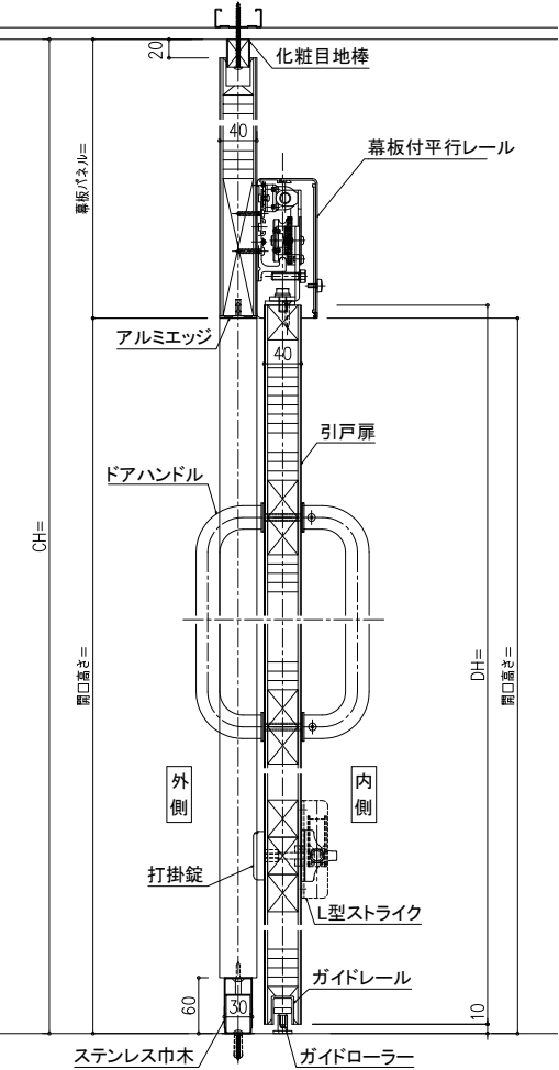
縦断面図_A
