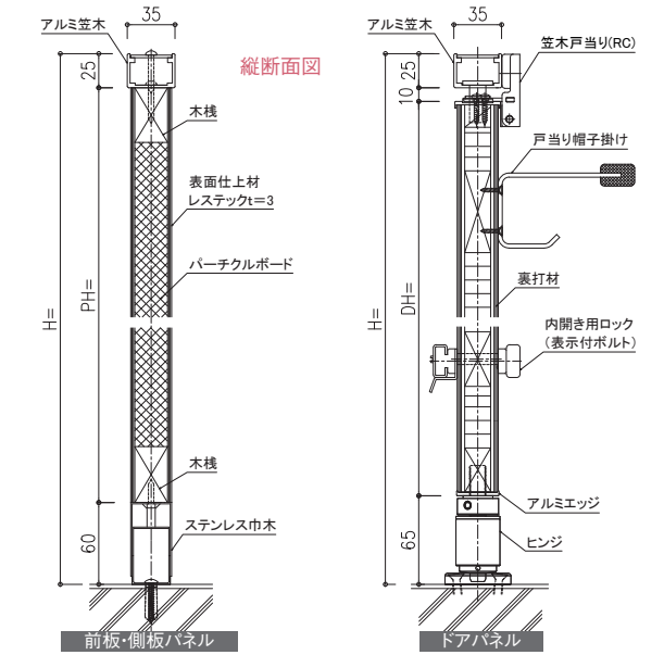
標準施工図例 UV-30RC
