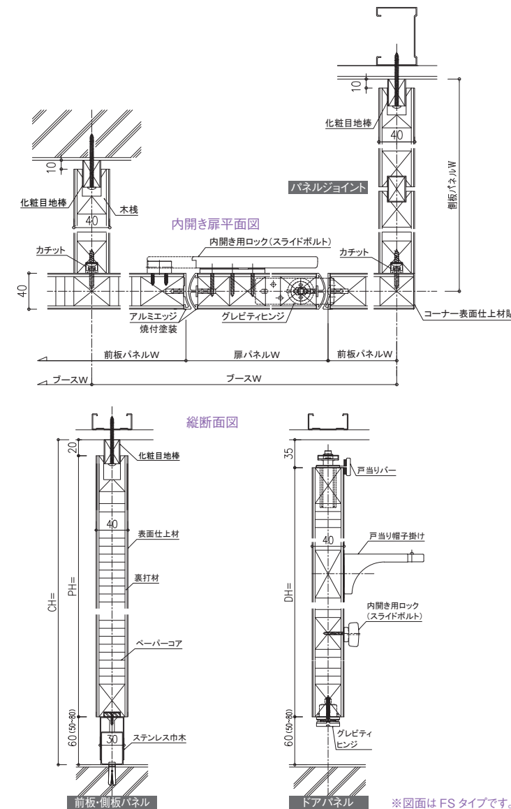
標準施工図例
