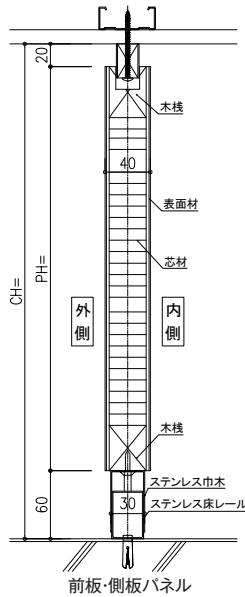
縦断面図_A
