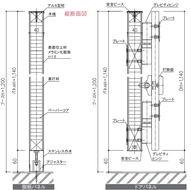
標準施工図例
