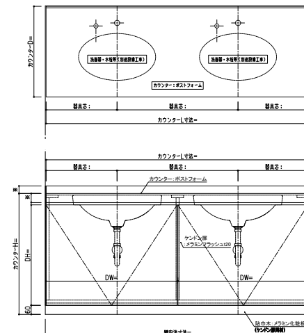
独立ボウルを配した、標準的なケन्दン扉仕様。
