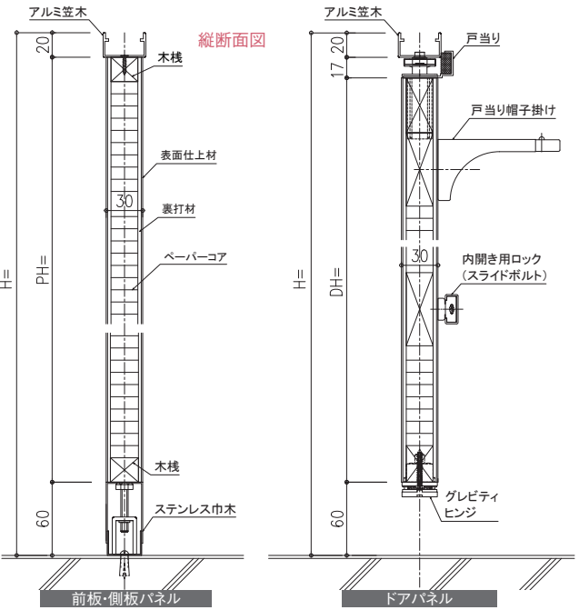
端部詳細図
