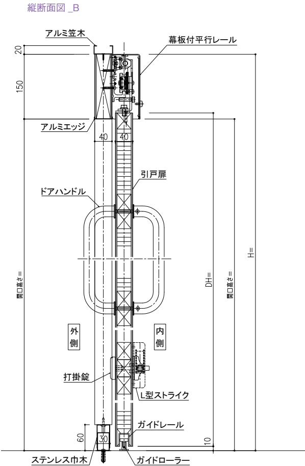
縦断面図_B
