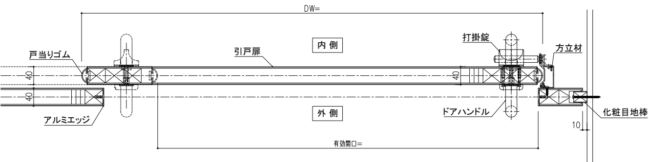
横断面図
