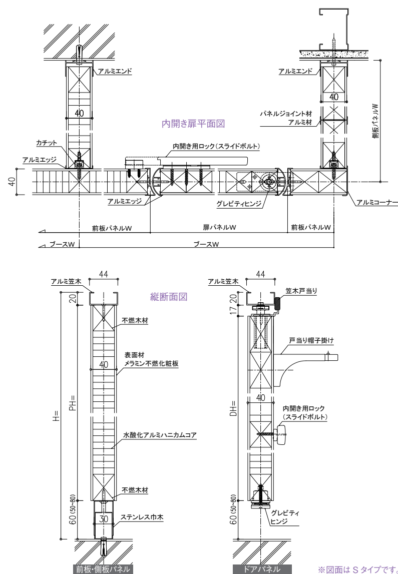
標準施工図例
