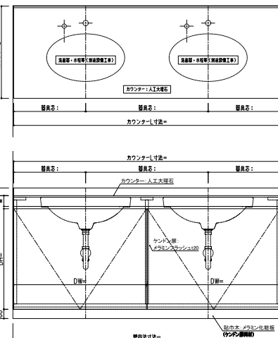
独立ボウルの、シンプルなケन्दン扉仕様。
